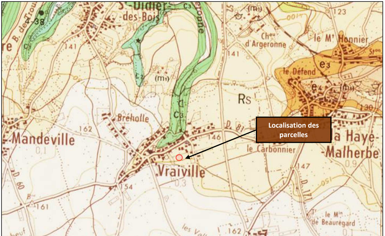
Extrait de la carte géologique au 1/25000
